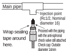
A-2. ATCF type
