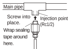
A-4. VTCET type
